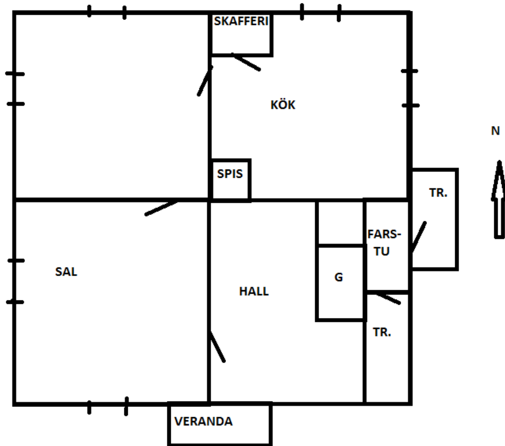
Planritning för botten våningen.
